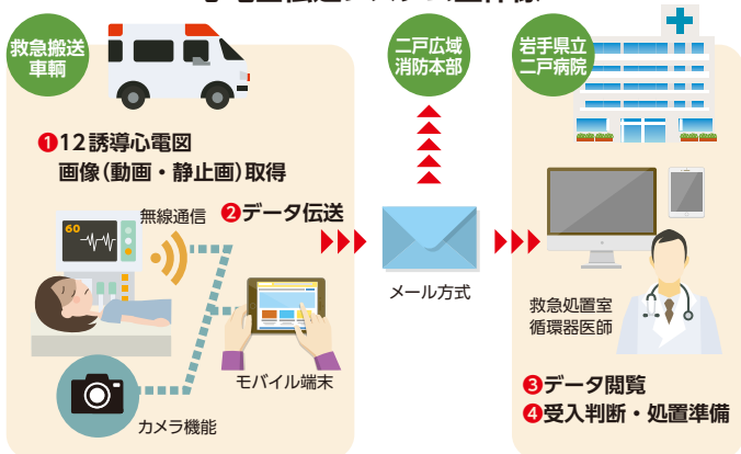
心電図伝送システム全体像
