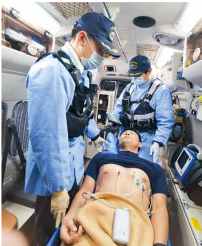
心電図伝送システム全体像
