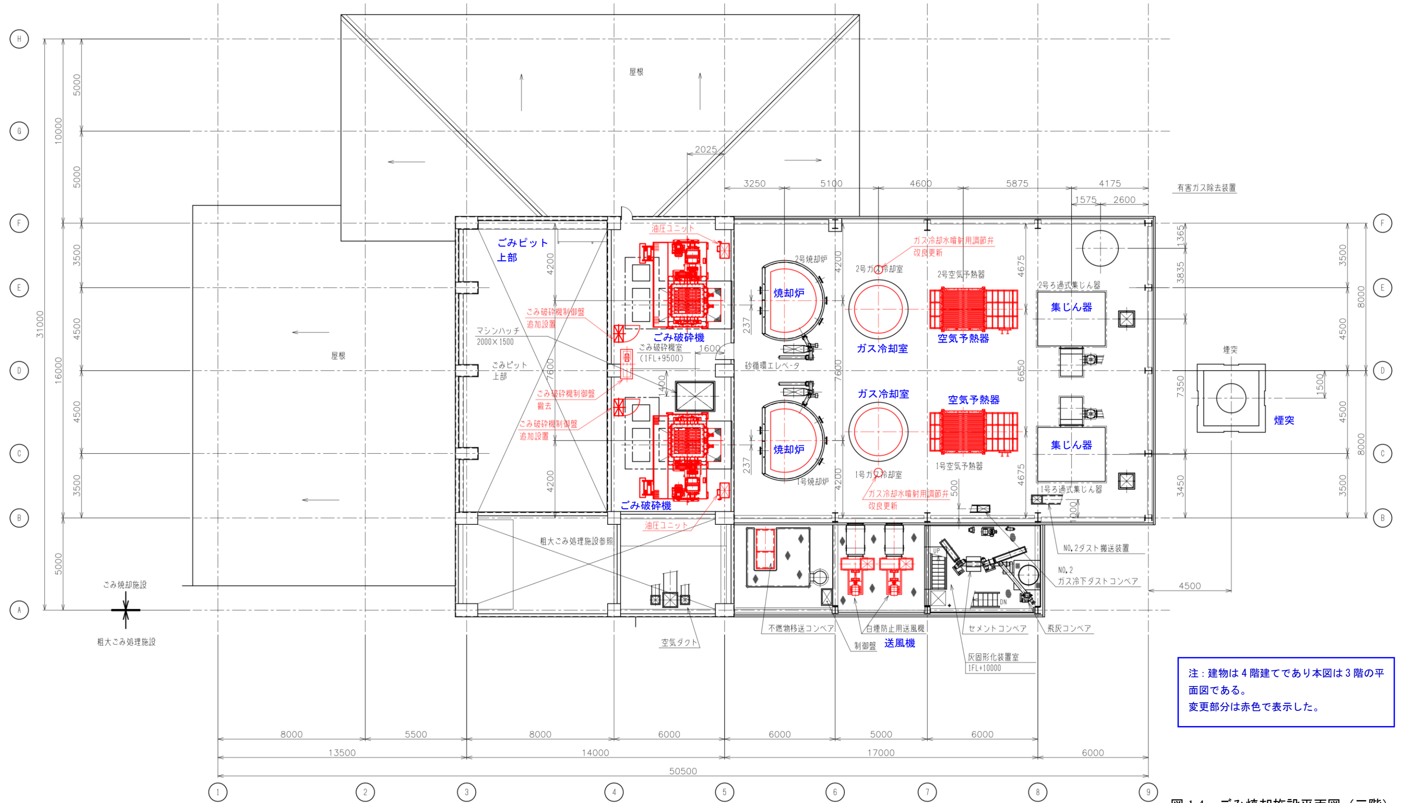
図 1.4 ごみ焼却施設平面図（三階）
